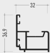
1 Telaio
