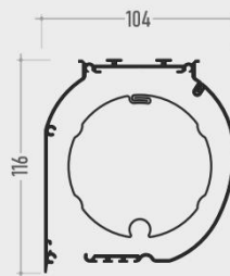
3 Scatola da 104 mm Albero \varnothing 78mm
