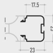
Guida inferiore a due foglie con estensione Centrale
