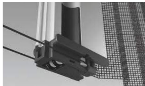
Due pulegge laterali, destra e sinistra, e rullo scorrevole con inserti in silicone
