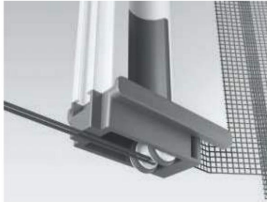
Puleggia inferiore con inserti in silicone
