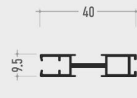
3 Guida scorrevole
