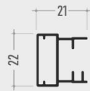
1 Ritenzione Guida
