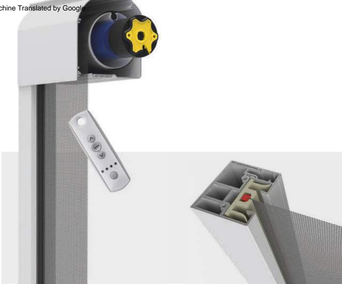
Sistema di ritenzione del tessuto ZIP
