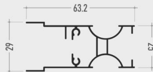
Guida laterale
