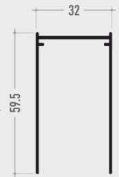
5 Sbarra
