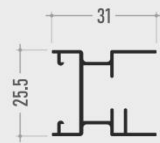
1 Ritenzione Guida
