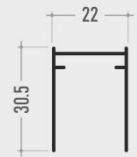
5 Sbarra
