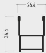
1 Perimetrale Guida
