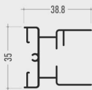
1 Ritenzione Guida
