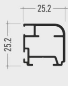
2 Foglia
