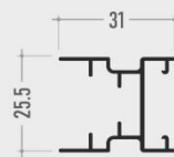
3 Guida laterale
