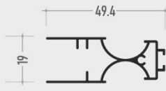
2 Guida scorrevole
