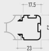
3 Bifoglia Scorrevole Estensione
