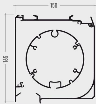
1 Scatola da 150 mm Albero \varnothing 110mm
