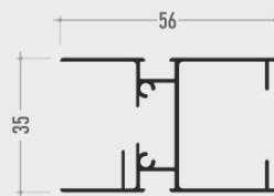
2 Guida scorrevole
