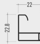
6 Soglia della porta R=1:2
