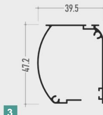
3 Scatola da 39 mm Installato esternamente o sotto il telaio
