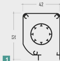
1 Scatola da 42 mm Lancia
