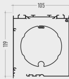
2 Scatola da 105 mm Albero \varnothing 78mm
