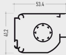
1 Scatola
