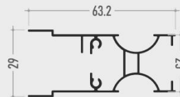
2 Guida scorrevole
