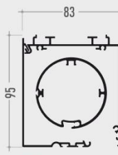
4 Scatola da 83 mm Albero \varnothing 60mm
