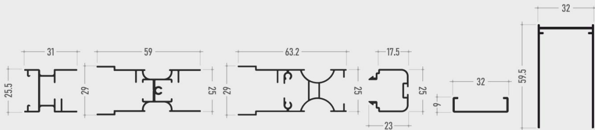
1 Ritenzione Guida
