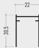
3 Laterale Guida OPALIO
