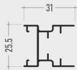
Guida laterale
