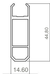
■ 360001 PROFILO AL. CURVO ALLUMINIO PROFILO CURVA
