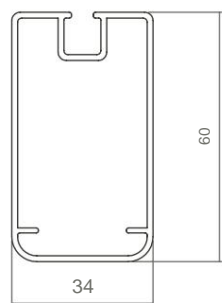
■ 320903 PROFILO DEL DADO DI CONTROLLO IN ALLUMINIO
