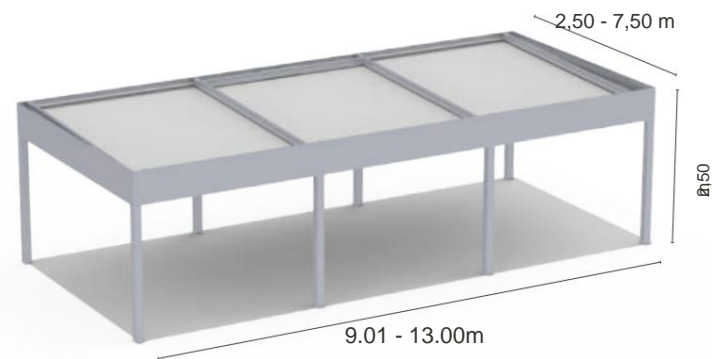
FLOPER 140 TELAIO DRIVER A 4 GUIDE FLOPER 140 TELAIO AUTOPORTANTE CON 4 GUIDE
