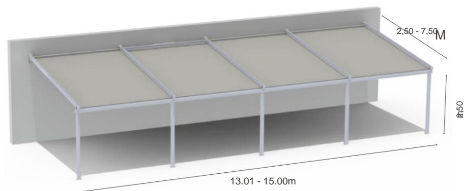
FLOPER 140 CON RINFORZO A 5 GUIDE FLOPER 140 CON GRONDAIA CON 5 GUIDE
