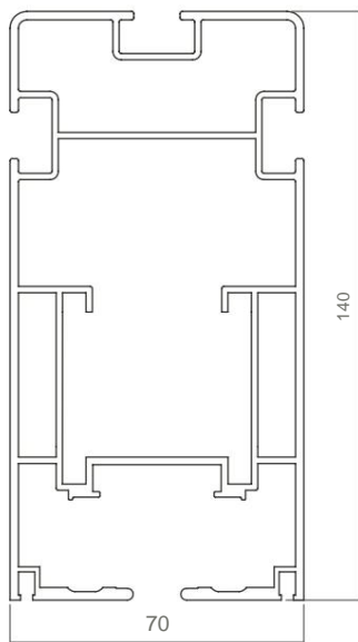
■ 327901 GUIDA FLOPER 140 FLOPER 140 GUIDA
