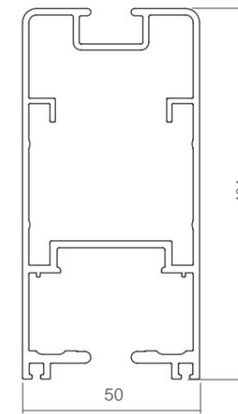
■ 320901 GUIDA FLOPER 100 GUIDA FLOPER 100
