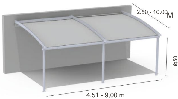
FLOPER 160 CURVA CON RINFORZO A 3 GUIDE FLOPER 160 CURVA CON GRONDA CON 3 GUIDE
