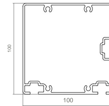
■ 325937 PROFILO SEZIONE TRAVERSA ALLUMINIO TRAVE LATERALE 100X100
