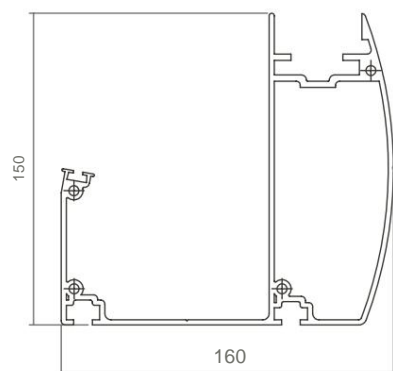
■ 325935 PROFILO DI DRENAGGIO IN ALLUMINIO GRONDAIA
