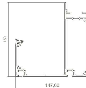
■ 325923 PROFILO AL. IDRO-FLUSSO RETTILINEO PROFILO IN ALLUMINIO GRONDAIA DI DRENAGGIO DRITTA
