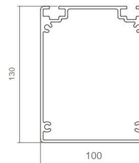
■ 325936 COLONNA IN PROFILO ALLUMINIO 130X100
