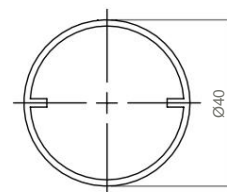
■ 320904 PROFILO ALLUMINIO TUBO F40 ALLUMINIO TUBO PROFILATO Ø40
