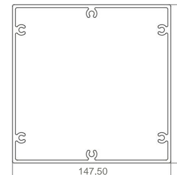
■ 328995 COLONNA IN PROFILO ALLUMINIO 150X150
