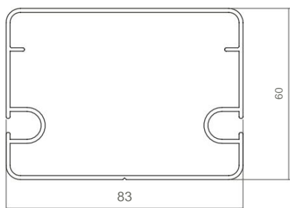
■ 320902 PROFILO ALTERNATIVO DEL CONTRAPPESO TERMINALE IN ALLUMINIO PROFILO DELLA BARRA
