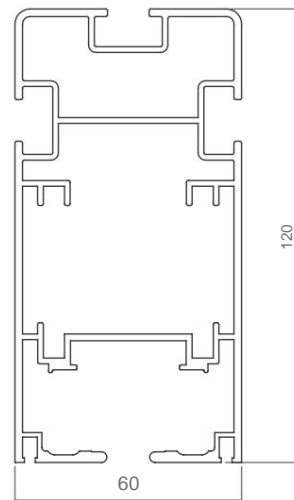
■ 322913 GUIDA FLOPER 120 FLOPER 120 GUIDA
